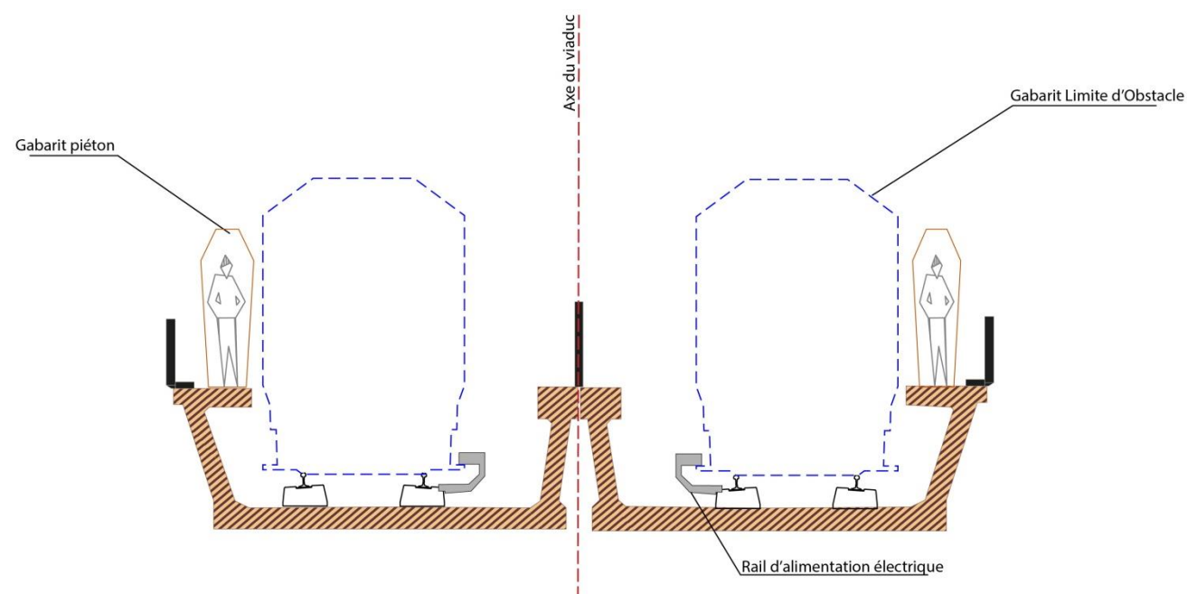
Exemple de coupe d'un viaduc en double petit U en alignement droit
