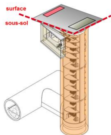
Exemple d'ouvrage relié au tunnel par un rameau
