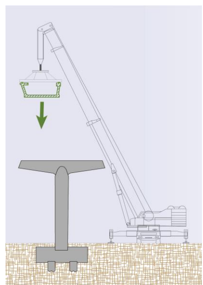
Principe de construction du viaduc (Société du Grand Paris)
